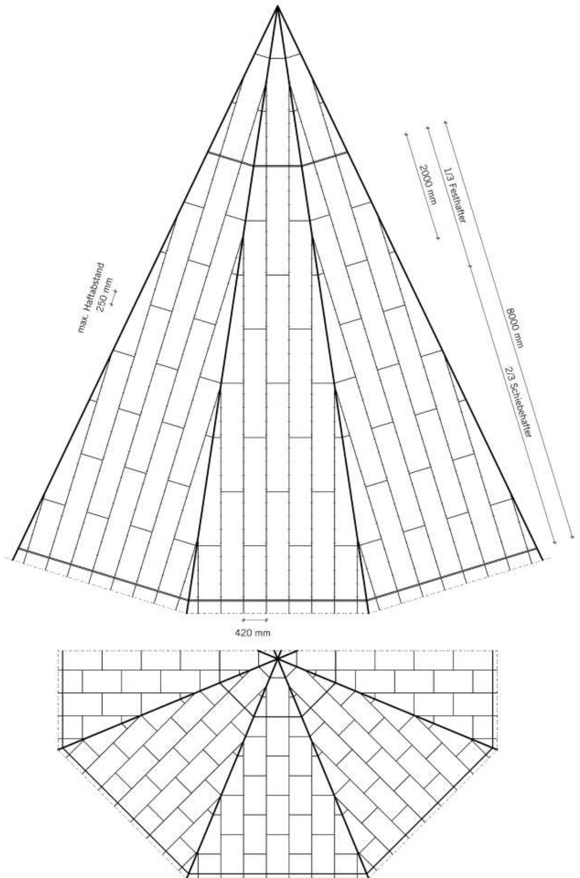
Abb. 6: Tafeldeckung als Bandverlegung ohne Befestigung der Querfalze
