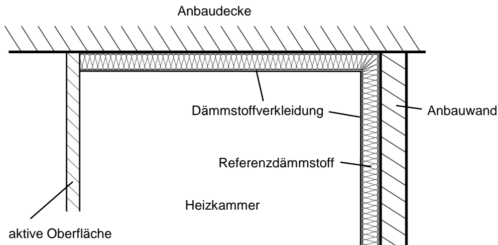
Abbildung 6.4.1-1: Beispiel für WDS 1: Referenzdämmstoff an Anbauflächen (Decke und Wand)
