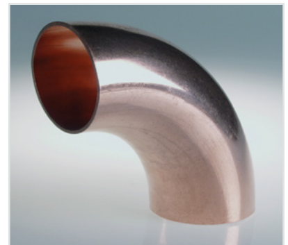
Bild 2.7 Schweißbogen DIN 2607 (5448)
